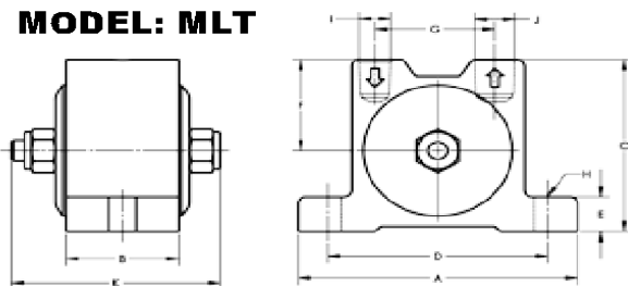
MODEL: MLT
